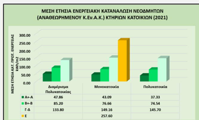
Γράφημα 17. Μέση ετήσια ενεργειακή κατανάλωση (kWh/m 2 ) νεόδμητων (αναθεωρημένου Κ.ΕΝ.Α.Κ.) κτηρίων κατοικιών (2021)
