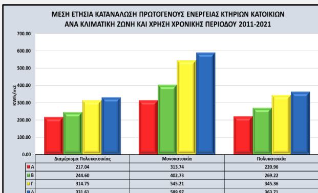
Γράφημα 43. Μέση ετήσια κατανάλωση πρωτογενούς ενέργειας κτηρίων κατοικιών ανά κλιματική ζώνη και χρήση (2011 – 2021).
