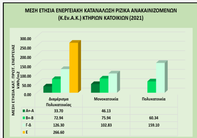
Γράφημα 11. Μέση ετήσια ενεργειακή κατανάλωση ( \text{kWh/m}^2 ) ριζικά ανακαινιζόμενων (Κ.Εν.Α.Κ.) κτηρίων κατοικιών (2021).
