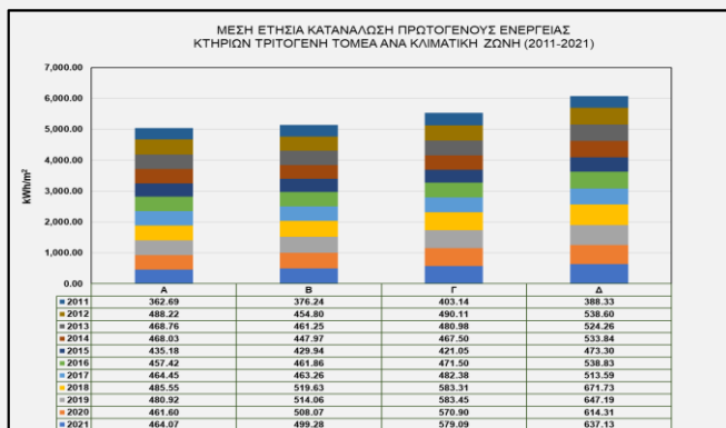
Γράφημα 50. Μέση ετήσια κατανάλωση πρωτογενούς ενέργειας κτηρίων τριτογενούς τομέα ανά κλιματική ζώνη και έτος (2011-2021).
