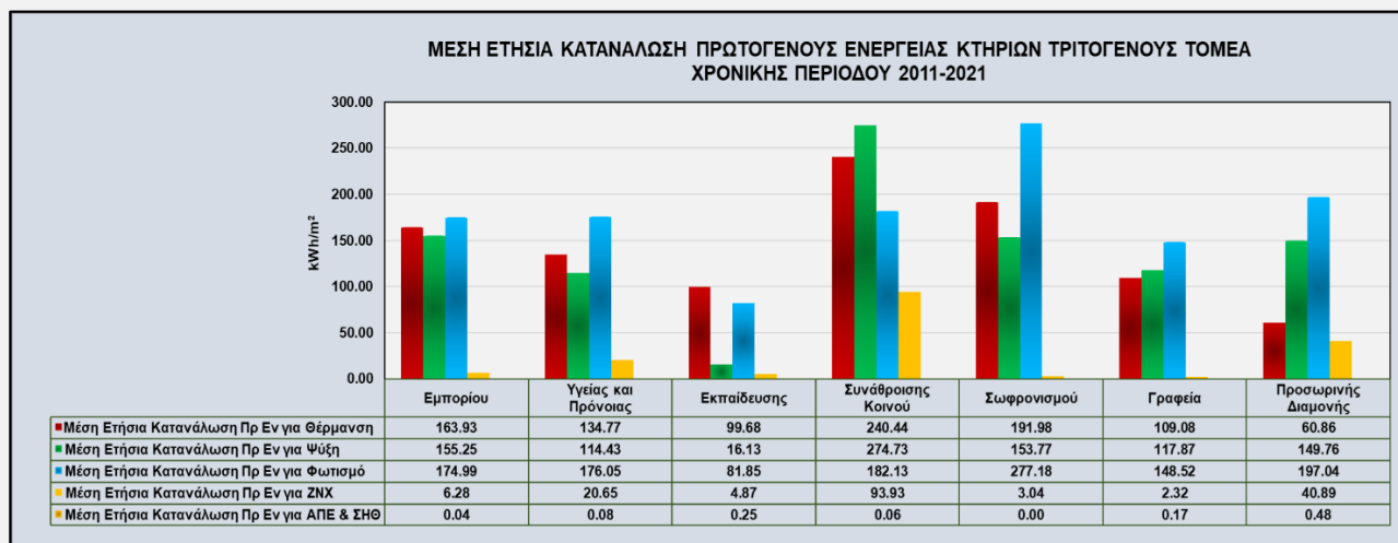
Γράφημα 49. Μέση ετήσια κατανάλωση πρωτογενούς ενέργειας κτηρίων τριτογενούς τομέα (2011-2021)
