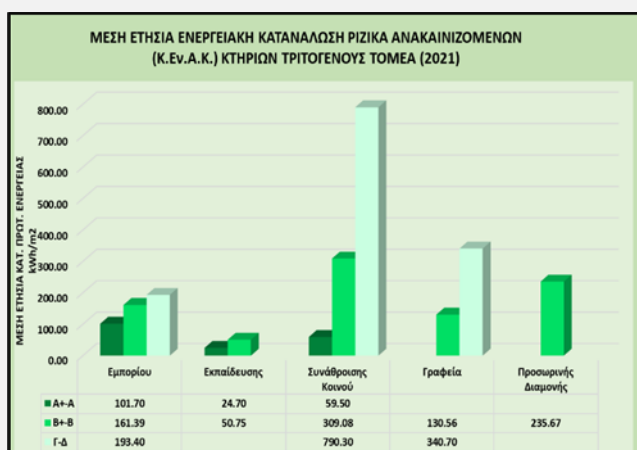
Γράφημα 13. Μέση ετήσια ενεργειακή κατανάλωση ( \text{kWh/m}^2 ) ριζικά ανακαινιζόμενων (Κ.Εν.Α.Κ.) κτηρίων τριτογενούς τομέα (2021).
