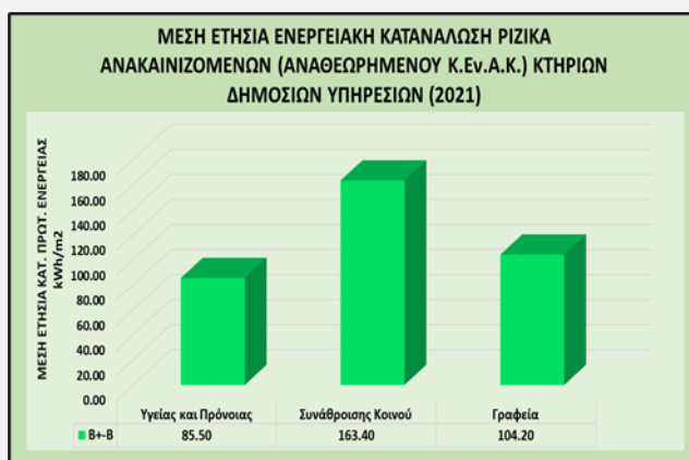
Γράφημα 27. Μέση ετήσια ενεργειακή κατανάλωση ριζικά ανακαινιζόμενων (αναθεωρημένου Κ.Εν.Α.Κ.) κτηρίων δημόσιων υπηρεσιών (2021).
