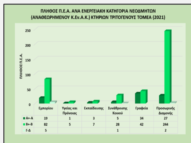
Γράφημα 20. Πλήθος Π.Ε.Α. ανά ενεργειακή κατηγορία νεόδμητων (αναθεωρημένου Κ.ΕΝ.Α.Κ.) κτηρίων τριτογενούς τομέα (2021).
