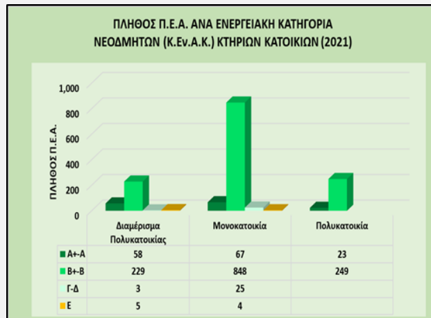
Γράφημα 6. Πλήθος Π.Ε.Α. ανά ενεργειακή κατηγορία νεόδμητων (Κ.Εν.Α.Κ.) κτηρίων κατοικιών (2021).
