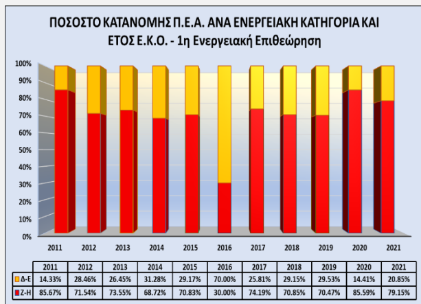
Γράφημα 81. Ποσοστό κατανομής Π.Ε.Α. ανά ενεργειακή κατηγορία και έτος για το πρόγραμμα «Εξοικονόμηση κατ' οίκον-Ι, Ι, ΙΙ, ΙΙb, Εξοικονομώ – Αυτονομώ 2020, Εξοικονομώ 2021» (1 η ενεργειακή επιθεώρηση).
