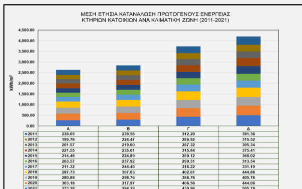
Γράφημα 42. Μέση ετήσια κατανάλωση πρωτογενούς ενέργειας κτηρίων κατοικιών ανά κλιματική ζώνη και έτος (2011 – 2021).
