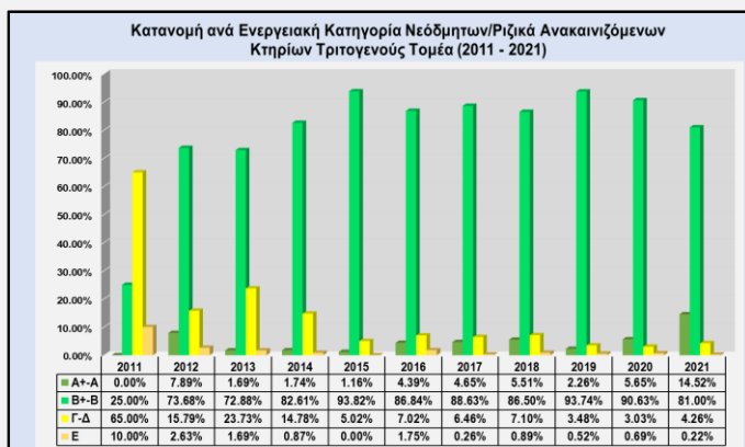
Γράφημα 69. Κατανομή ανά ενεργειακή κατηγορία νεόδμητων / ριζικά ανακαινιζόμενων κτηρίων τριτογενούς τομέα (2011-2021).
