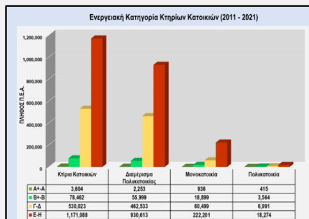
Γράφημα 40. Ενεργειακή κατηγορία κτηρίων κατοικιών (2011-2021).
