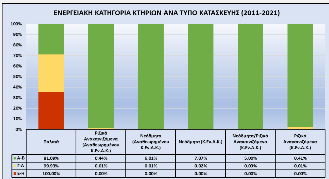
Γράφημα 31. Ενεργειακή Κατηγορία Κτηρίων ανά τύπο κατασκευής (2011 – 2021).
