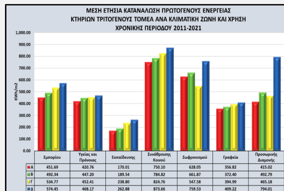
Γράφημα 51. Μέση ετήσια κατανάλωση πρωτογενούς ενέργειας κτηρίων τριτογενούς τομέα ανά κλιματική ζώνη και χρήση (2011 - 2021).
