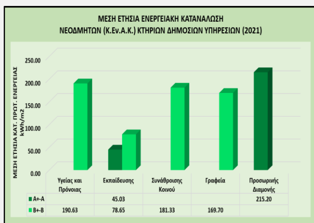
Γράφημα 9. Μέση ετήσια ενεργειακή κατανάλωση (kWh/m 2 ) νεόδμητων (Κ.Εν.Α.Κ.) κτηρίων δημόσιων υπηρεσιών (2021).
