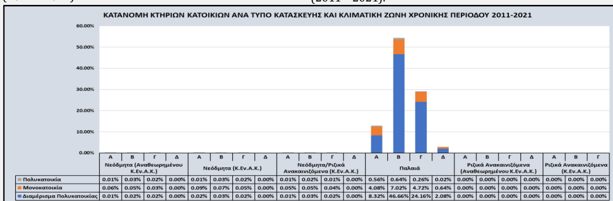
Γράφημα 44. Κατανομή κτηρίων κατοικιών ανά τύπο κατασκευής και κλιματική ζώνη (2011-2021).
