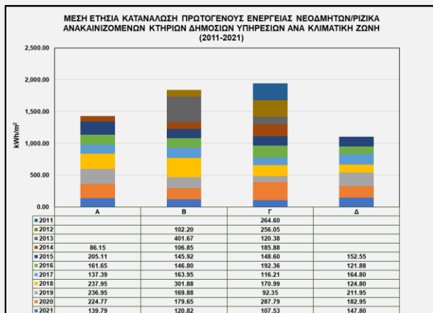
Γράφημα 78. Μέση ετήσια κατανάλωση πρωτογενούς ενέργειας νεόδμητων/ριζικά ανακαινιζόμενων κτηρίων δημόσιων υπηρεσιών ανά κλιματική ζώνη και έτος (2011-2021).
