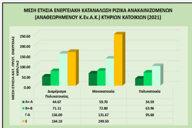
Γράφημα 23. Μέση ετήσια ενεργειακή κατανάλωση ριζικά ανακαινιζόμενων (αναθεωρημένου Κ.Εν.Α.Κ.) κτηρίων κατοικιών (2021).
