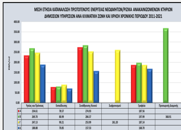
Γράφημα 79. Μέση ετήσια κατανάλωση πρωτογενούς ενέργειας νεόδμητων/ριζικά ανακαινιζόμενων κτηρίων δημόσιων υπηρεσιών ανά κλιματική ζώνη και χρήση (2011-2021).
