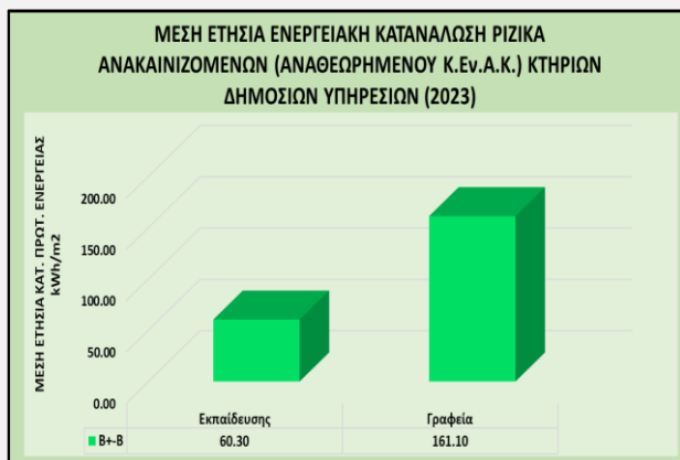
Γράφημα 27. Μέση ετήσια ενεργειακή κατανάλωση ριζικά ανακαινιζόμενων (αναθεωρημένου Κ.Εν.Α.Κ.) κτηρίων δημόσιων υπηρεσιών (2023).
