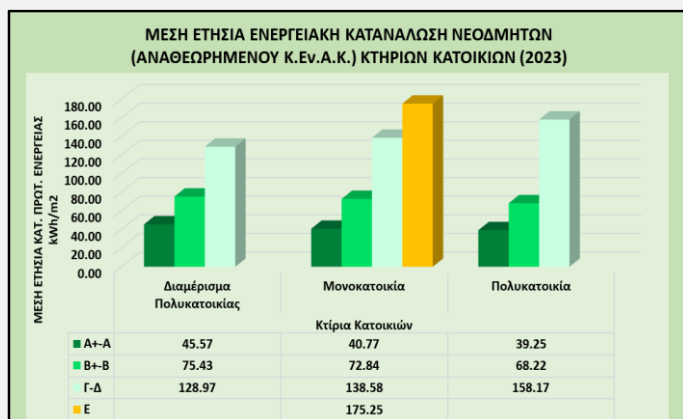
Γράφημα 17. Μέση ετήσια ενεργειακή κατανάλωση (kWh/m 2 ) νεόδμητων (αναθεωρημένου Κ.Εν.Α.Κ.) κτηρίων κατοικιών (2023).
