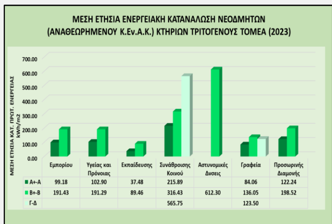
Γράφημα 19. Μέση ετήσια ενεργειακή κατανάλωση (kWh/m 2 ) νεόδμητων (αναθεωρημένου Κ.Εν.Α.Κ.) κτηρίων τριτογενούς τομέα (2023).
