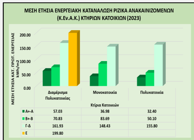
Γράφημα 11. Μέση ετήσια ενεργειακή κατανάλωση (kWh/m²) ριζικά ανακαινιζόμενων (Κ.ΕΝ.Α.Κ.) κτηρίων κατοικιών (2023).
