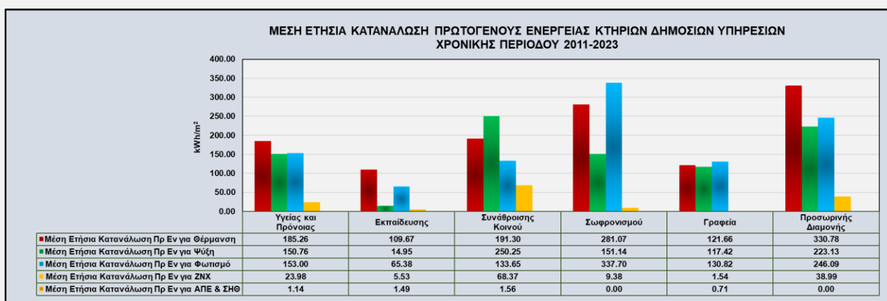
Γράφημα 57. Μέση ετήσια κατανάλωση πρωτογενούς ενέργειας κτηρίων δημόσιων υπηρεσιών (2011-2023).
