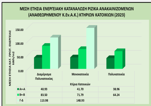
Γράφημα 23. Μέση ετήσια ενεργειακή κατανάλωση ριζικά ανακαινιζόμενων (αναθεωρημένου Κ.Εν.Α.Κ.) κτηρίων κατοικιών (2023).
