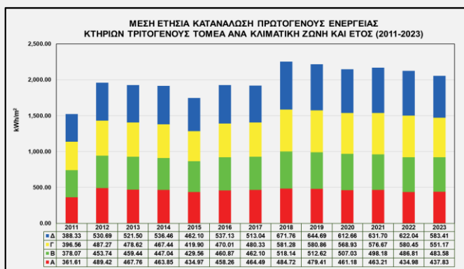
Γράφημα 50. Μέση ετήσια κατανάλωση πρωτογενούς ενέργειας κτηρίων τριτογενούς τομέα ανά κλιματική ζώνη και έτος (2011-2023).
