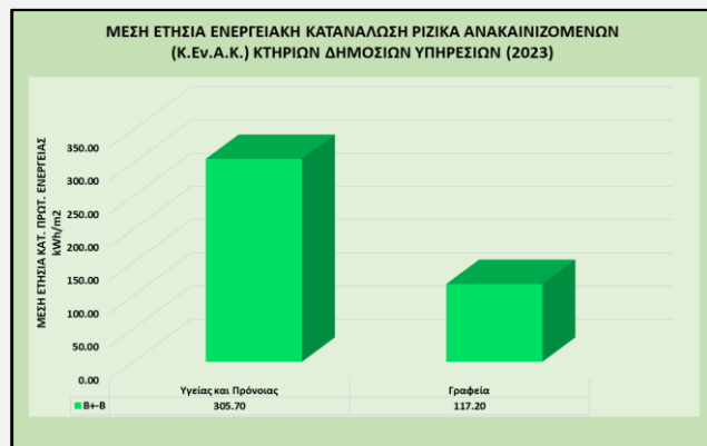
Γράφημα 15. Μέση ετήσια ενεργειακή κατανάλωση (kWh/m²) ριζικά ανακαινιζόμενων (Κ.ΕΝ.Α.Κ.) κτηρίων δημόσιων υπηρεσιών (2023).
