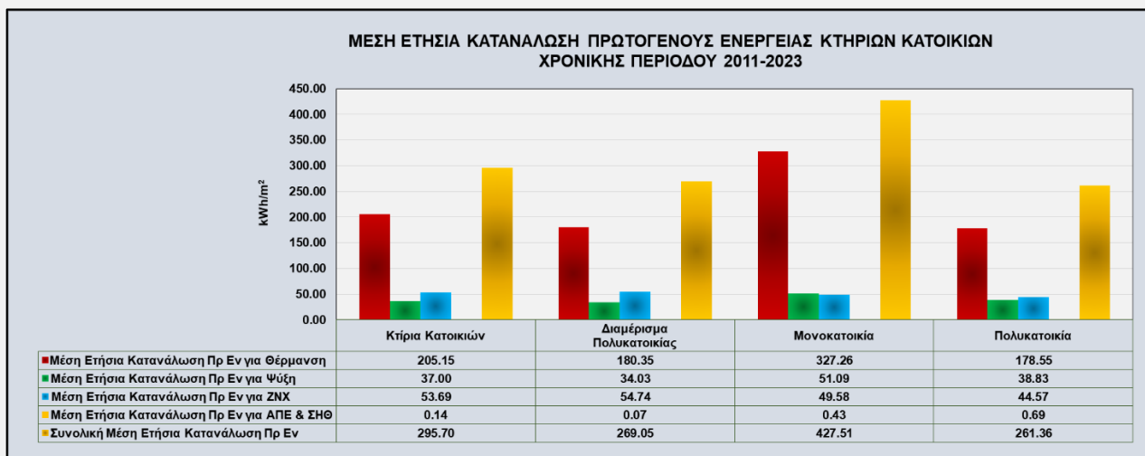
Γράφημα 41. Μέση ετήσια κατανάλωση πρωτογενούς ενέργειας κτηρίων κατοικιών (2011-2023).
